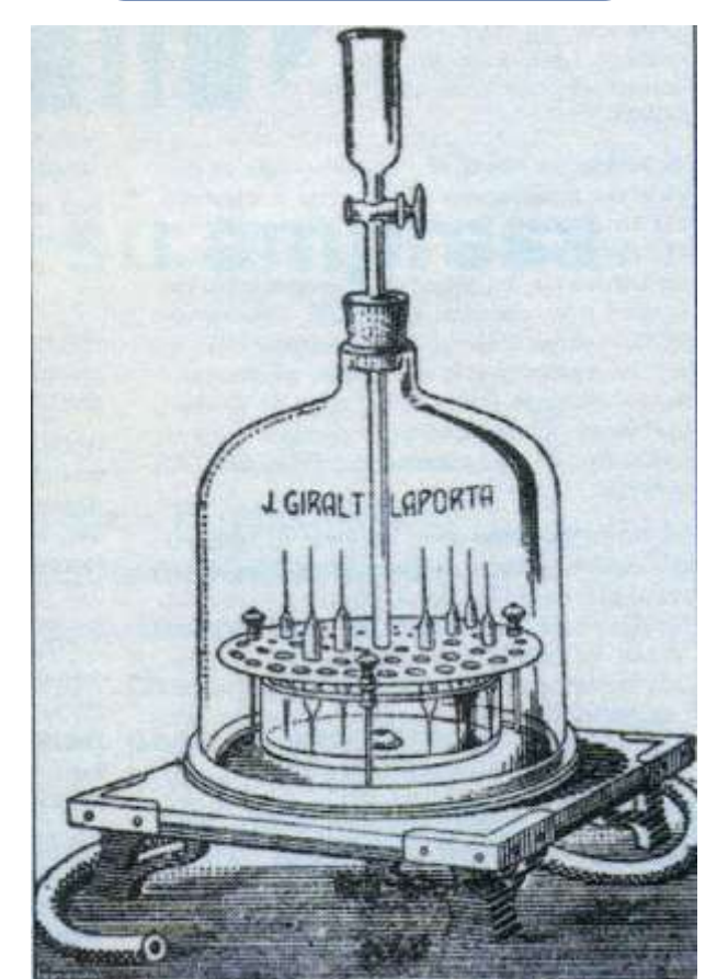
Aparato de llenado de ampollas medicinales por medio del vacío, fabricado por J. Giralt Laporta.
